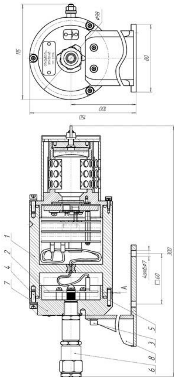
Рисунок А.1- Сборочный чертёж датчика ГСО-Р1Д.
